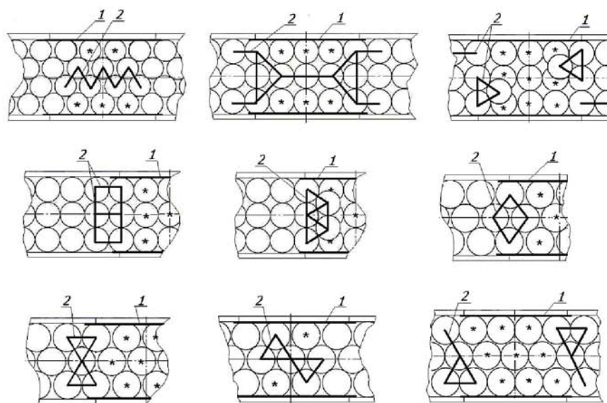
Рисунок 30 – Примеры размещения и увязки мягких контейнеров
