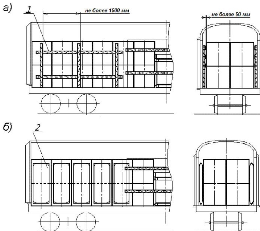
Рисунок 22 – Примеры крепления рулонов в поперечном направлении
