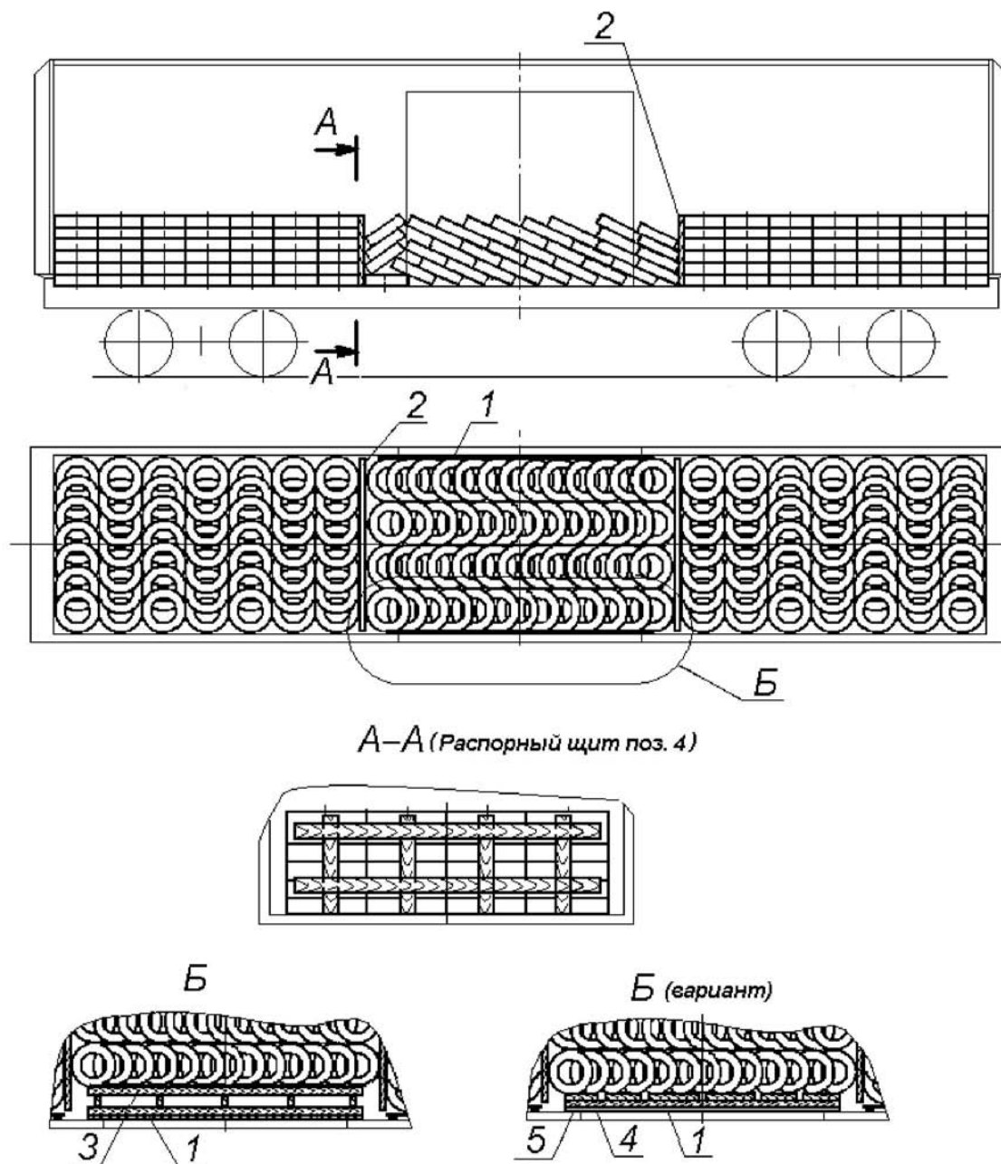
Рисунок 27 – Пример размещения бунтов в наклонном положении 1 – ограждение дверного проема; 2 – распорный щит; 3 – распорная рама; 4 – упорный брус; 5 – распорный брус
